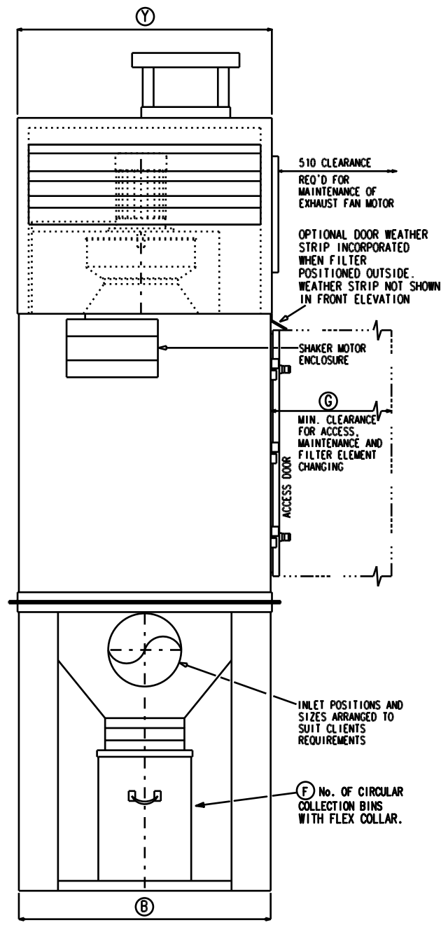
END ELEVATION
